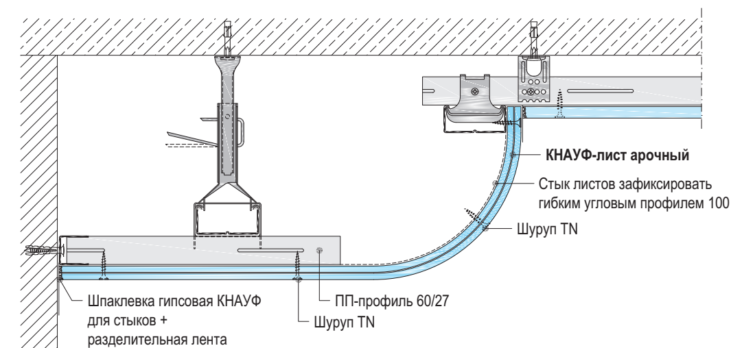
Гибкий угловой профиль
