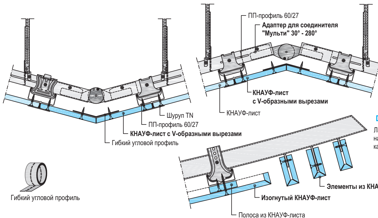
Зигзагообразный потолок П191.ru-S26A
