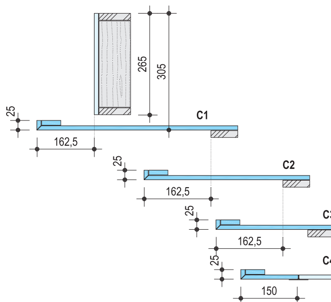
Сечение С-С
