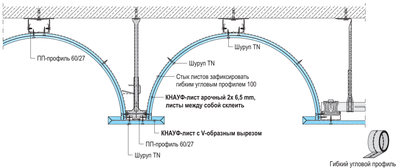
Схематические чертежи
