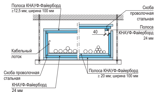
Схема бескаркасного кабельного короба
