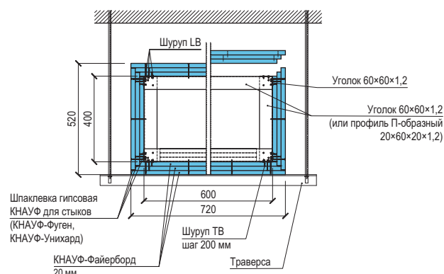
Схема каркасного кабельного короба
