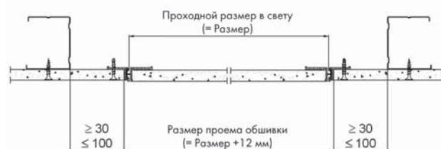
Схематический чертеж люка для помещений с повышенной влажностью
