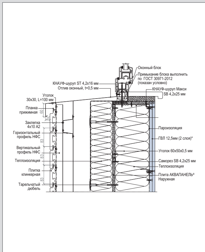
А 4 – WM 111 (4а 100) С. Нижнее примыкание к оконному блоку
