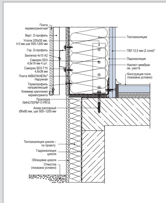
С 4 – WM 112 (2) С. Примыкание к фундаменту. Вариант 1
