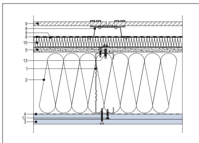
Рис. 8. Тип № 3. Схема конструктивного исполнения наружной несущей КОС с зазором с внешней стороны и дополнительным наружным утеплением (расшифровку цифровых обозначений см. в табл. 1)
