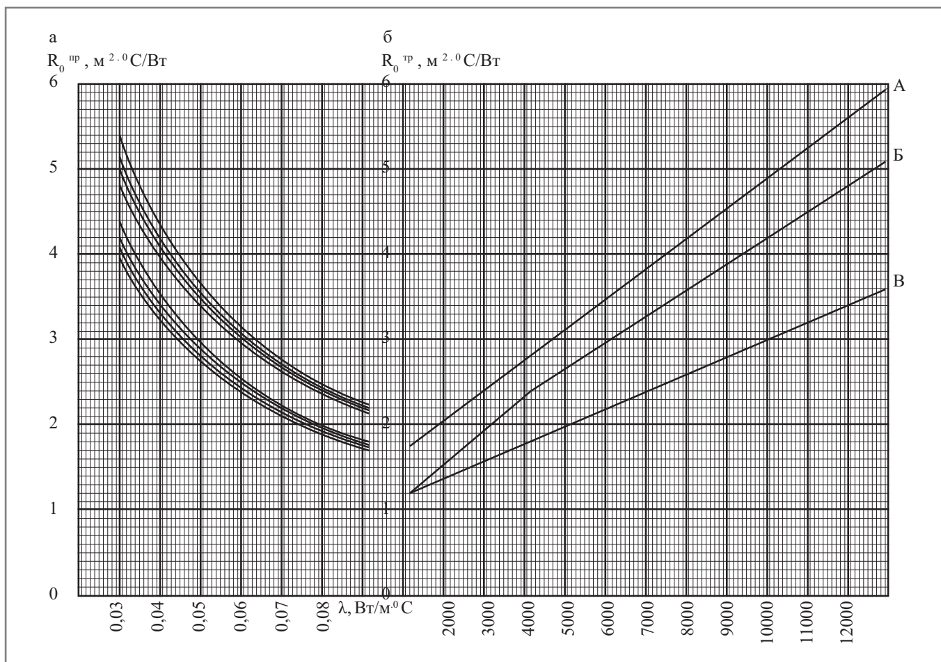
Рис. 15. Приведенное сопротивление теплопередаче стен ( R_0^{np} ) с каркасом из термопрофилей толщиной: 0,7 (1); 1,0 (2); 1,2 (3) и 1,5 (4) мм при толщине теплоизоляции 150 (I) и 200 (II) мм в зависимости от расчетного значения коэффициента теплопроводности теплоизоляции ( \lambda ) в сравнении с требуемыми ( R_0^{np} ) из условия энергосбережения значениями сопротивления теплопередаче наружных КОС с применением ЛСТК в зданиях: жилых (А), общественных (Б) и производственных (В), в зависимости от расчетных значений градусо-суток отопительного периода (ГСОП)
