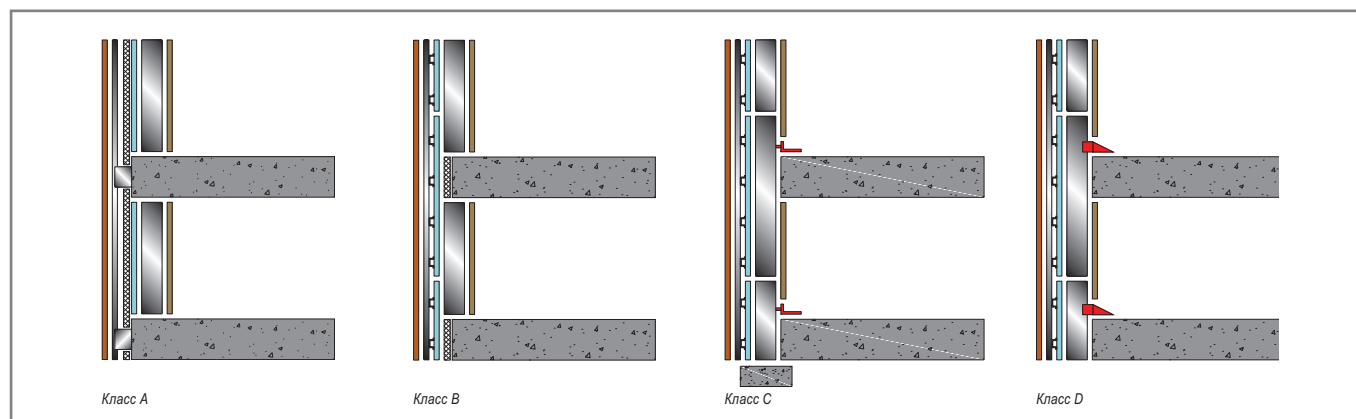
Рис. 5. Классификация наружных несущих стен в зависимости от типа примыкания к несущим конструкциям здания
