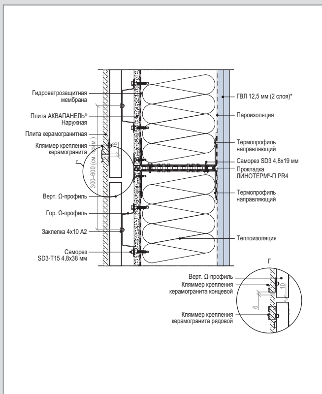
С 6 – WM 112 (2) С. Горизонтальный стык смежных модулей
