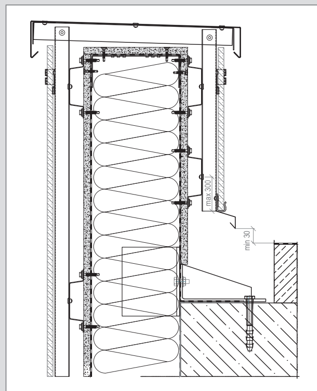
D 4 – WM 112 (2) C. Крепление к плите покрытия. Паралет
