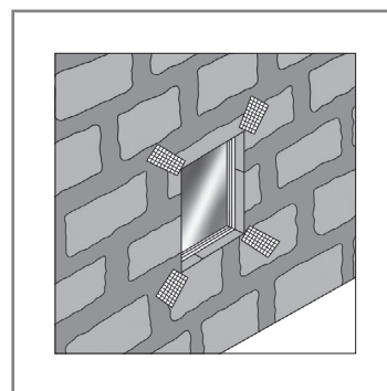
Рис. 29. Армирование обшивки в углах оконных и дверных проемов
