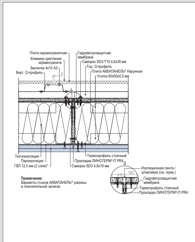
С 6 – WM 112 (2) С. Вертикальный стык смежных модулей
