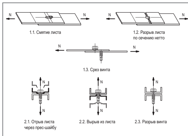
Рис. 12. Графическое изображение типов отказа соединений тонкостенных конструкций на саморезах
