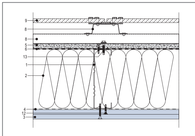
Рис. 7. Тип № 2. Схема конструктивного исполнения наружной несущей КОС с зазором с внешней стороны (расшифровку цифровых обозначений см. в табл. 1)
