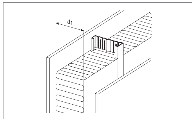
Рис. 14. Толщина утепляющего слоя наружной КОС с применением ЛСТК
