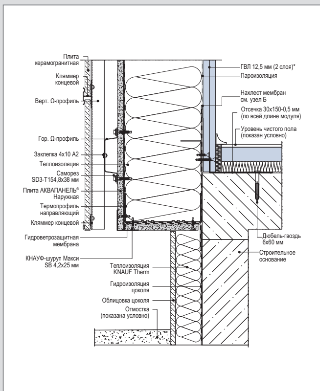
D 7 – WM 112 (2) С. Примыкание к фундаменту
