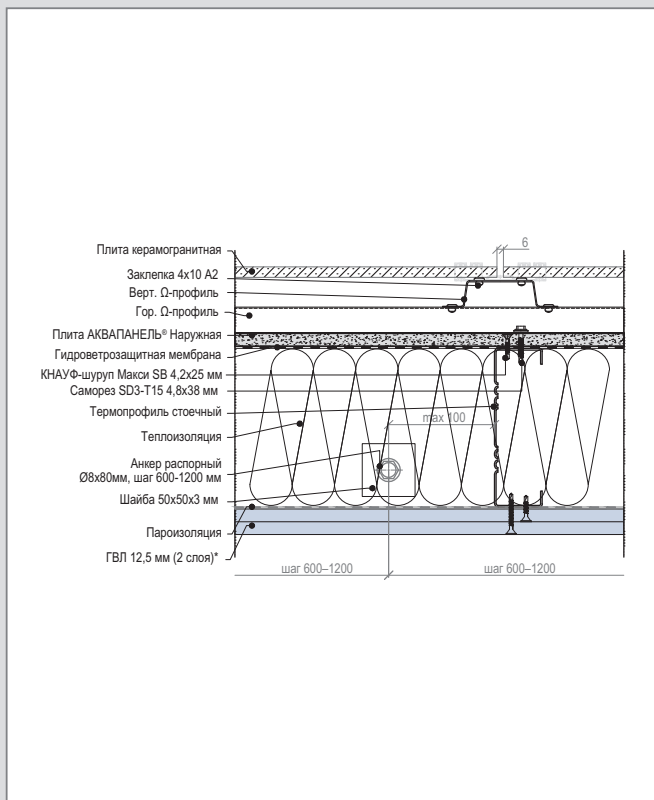
В 3 – WM 112 (2) С. Горизонтальный разрез рядового модуля. Примыкание к перекрытию. Вариант 1
