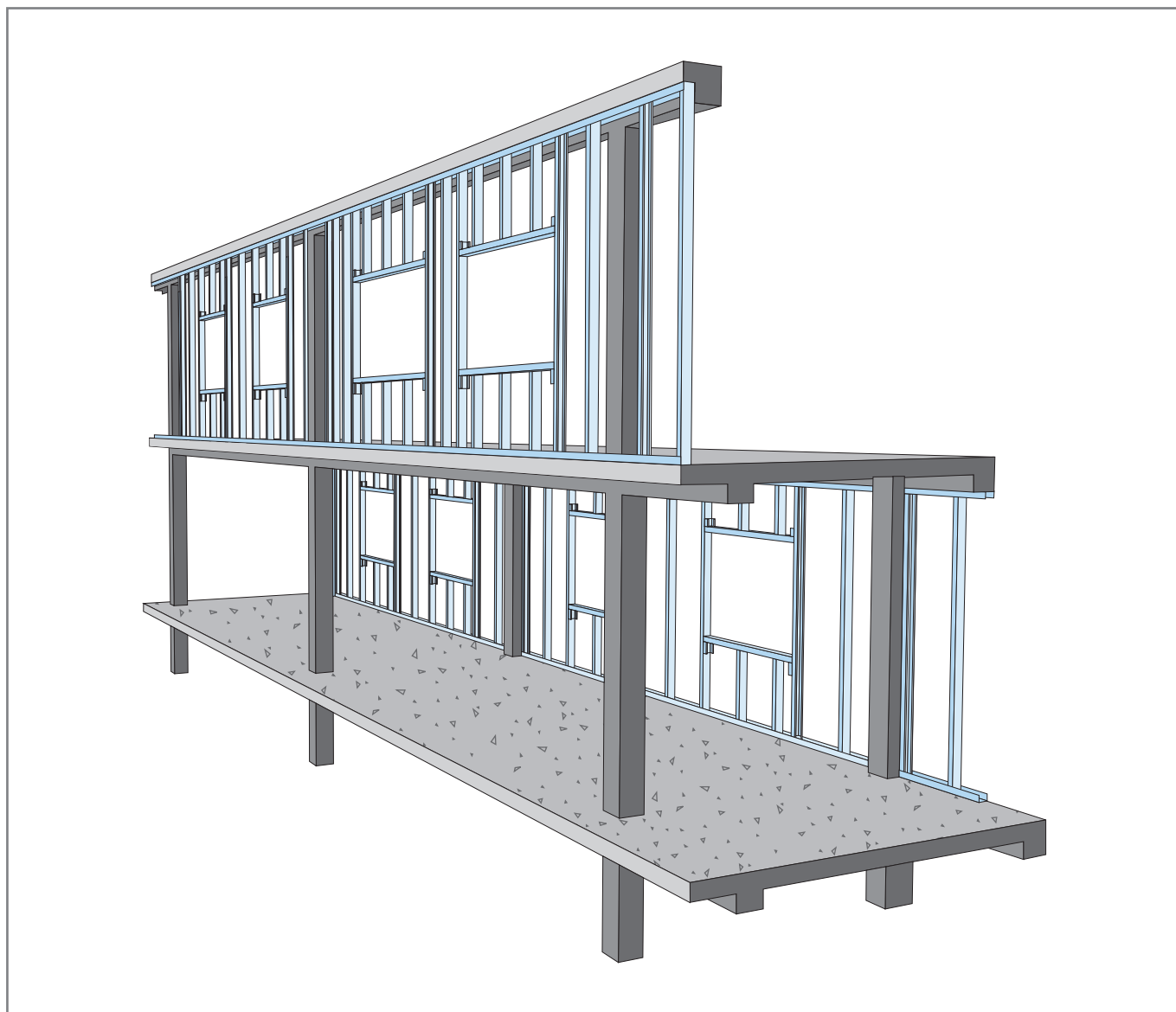
Рис. 3. Схематическое изображение несущих КОС с каркасом из ЛСТК (класс А или В) в здании с несущим монолитным железобетонным каркасом
