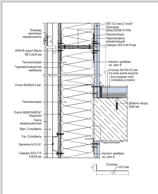
С 3 – WM 112 (2) С. Вертикальный разрез рядового модуля
