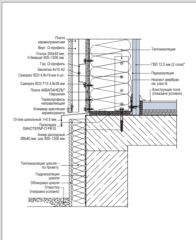
С 5 – WM 112 (2) С. Примыкание к фундаменту. Вариант 2
