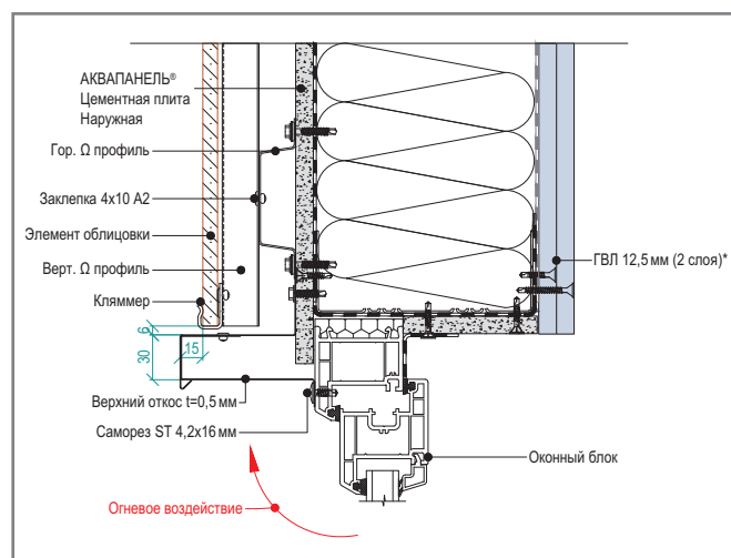
Рис. 8а. Пример узла верхнего откоса с противопожарной отсечкой пламени огня
