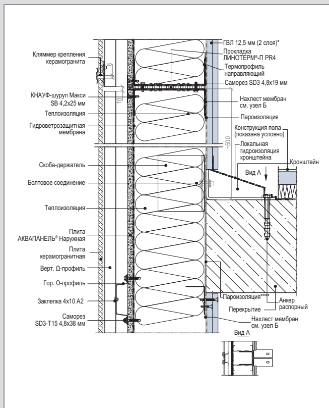
D 1 – WM 112 (2) C. Вертикальный разрез рядового модуля. Крепление к перекрытию
