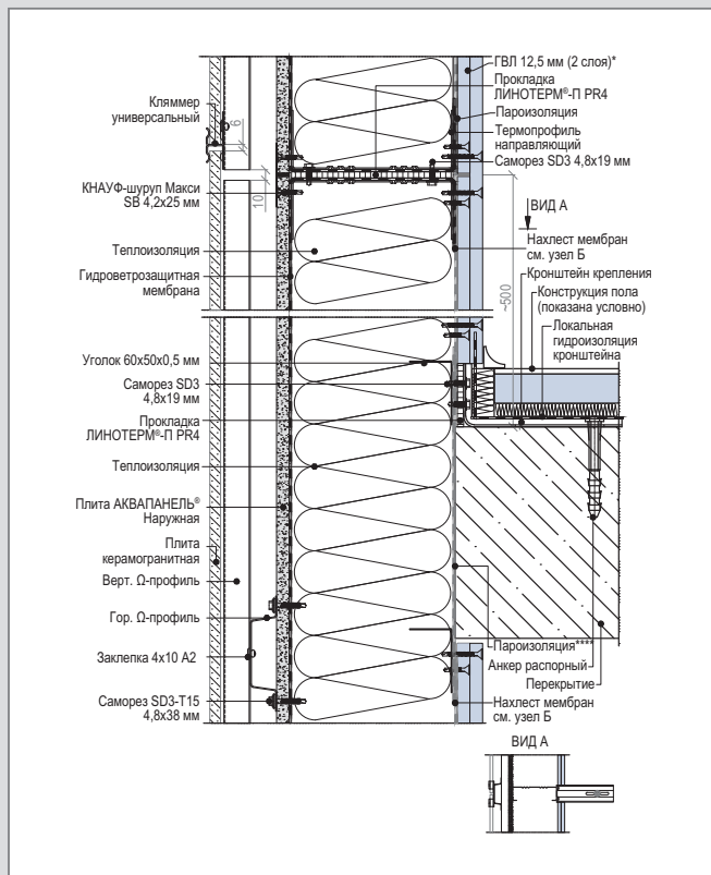
С 1 – WM 112 (2) С. Вертикальный разрез рядового модуля. Крепление к перекрытию
