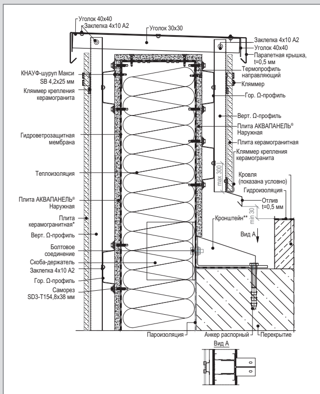
D 5 – WM 112 (2) С. Примыкание к плите покрытия
