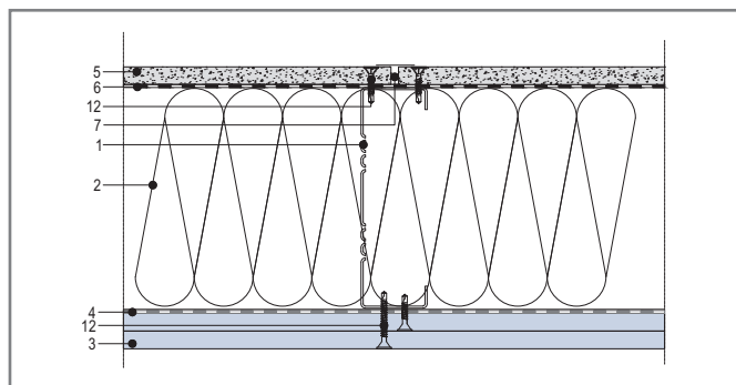
Рис. 6. Тип № 1. Схема конструктивного исполнения наружной несущей КОС без зазора с внешней стороны (расшифровку цифровых обозначений см. в табл. 1)
