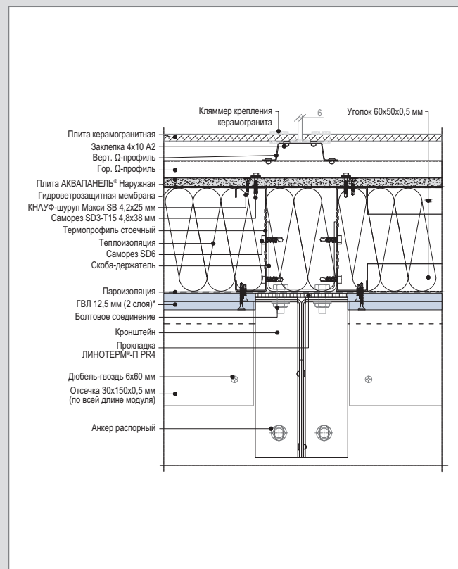
D 2 – WM 112 (2) C. Горизонтальный разрез рядового модуля. Крепление к перекрытию
