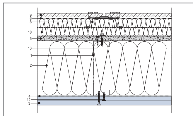
Рис. 9. Тип № 4. Схема конструктивного исполнения наружной несущей КОС с зазором и дополнительным наружным утеплением (расшифровку цифровых обозначений см. на рис. 2)
