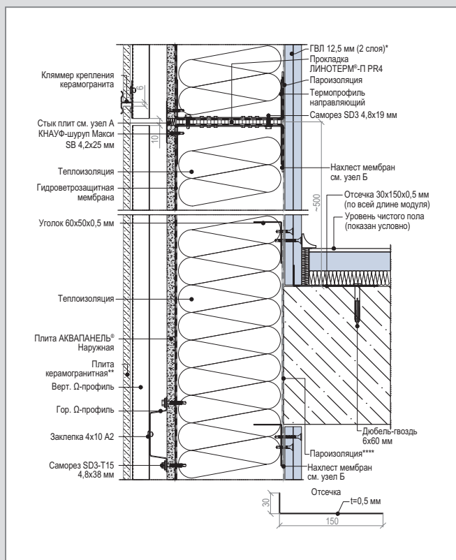
D 3 – WM 112 (2) C. Вертикальный разрез рядового модуля
