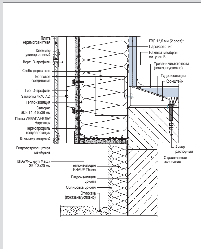
D 6 – WM 112 (2) С. Крепление к фундаменту
