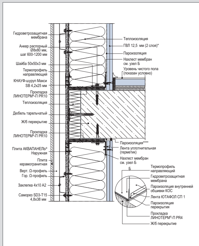
В 2 – WM 112 (2) С. Вертикальный разрез рядового модуля. Примыкание к перекрытию. Вариант 1
