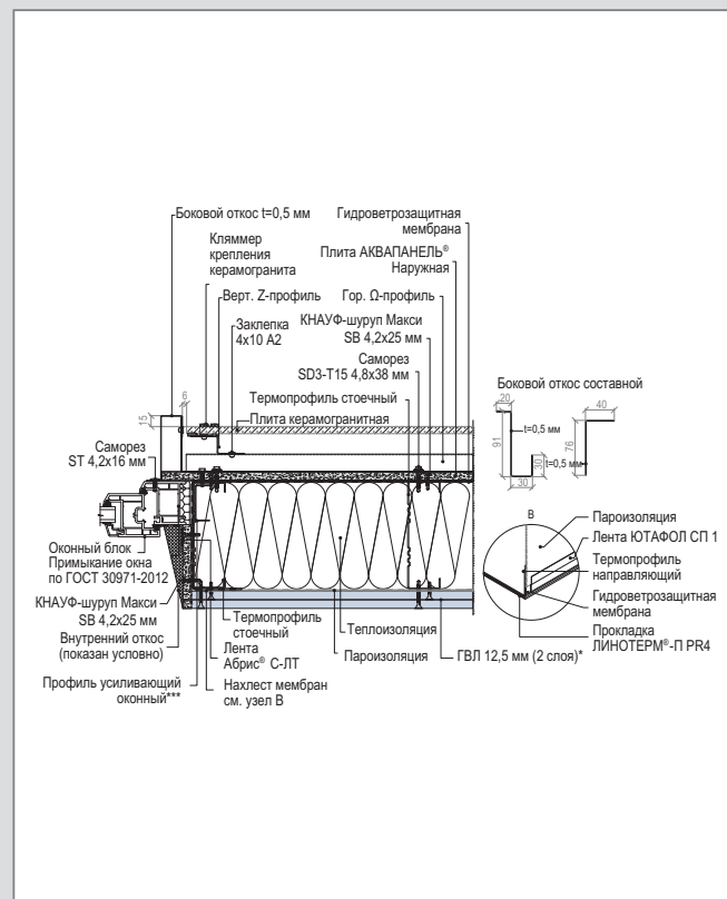
В 6 – WM 112 (2) С. Боковое примыкание к оконному блоку
