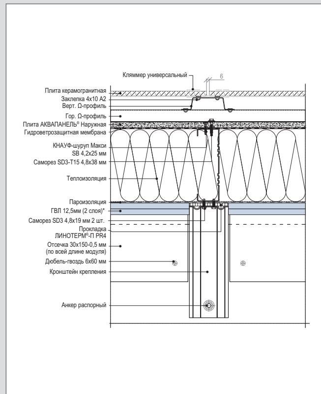
С 2 – WM 112 (2) С. Горизонтальный разрез рядового модуля. Крепление к перекрытию
