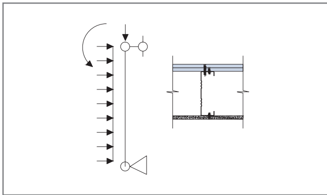
Рис. 11. Расчетная схема стойки каркаса стены при воздействии ветровой нагрузки и нагрузки от собственного веса фасада, схема раскрепления полок стойки термопрофиля обшивками КОС
