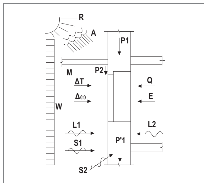
Рис. 10. Воздействия на наружные несущие КОС
