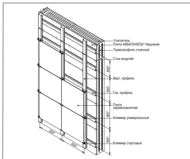
Рис. 1. Общий вид наружной каркасно-обшивной стены (КОС) с каркасом из ЛСТК
