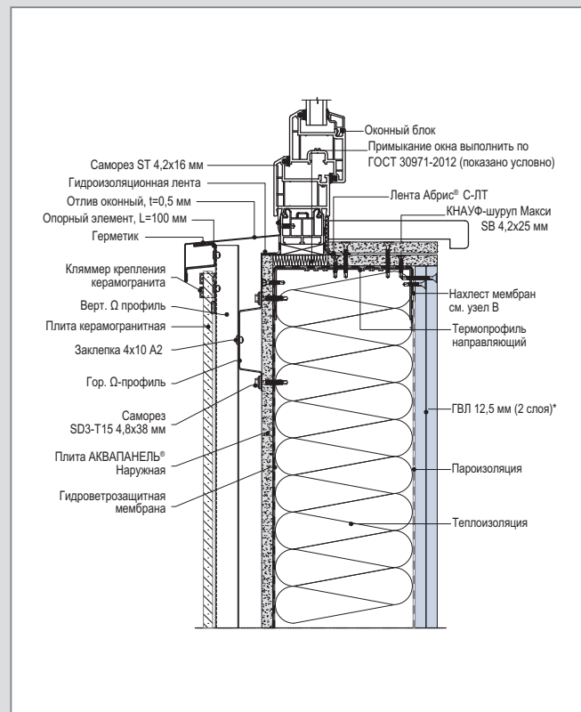
В 8 – WM 112 (2) С. Нижнее примыкание к оконному блоку
