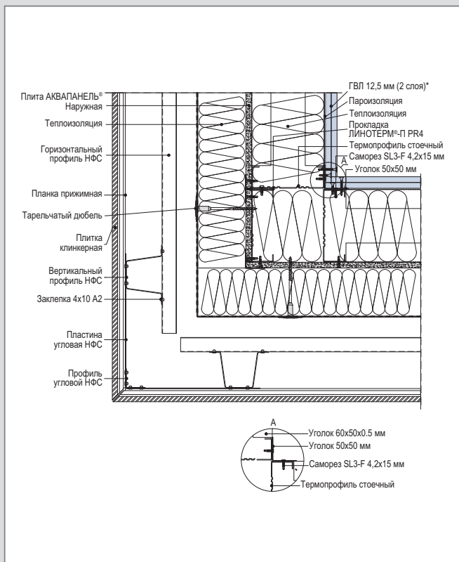
A 2 – WM 111 (4а 100) С. Горизонтальный разрез внешнего угла
