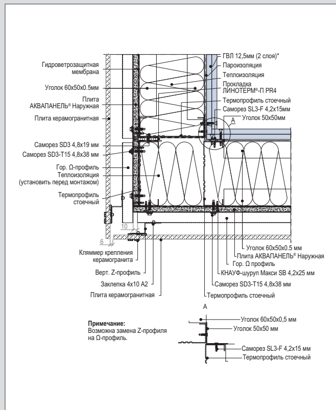
В 9 – WM 112 (2) С. Внешний угол
