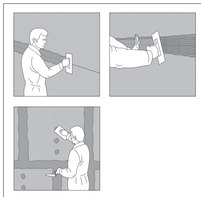
Рис. 24. Шпаклевание стыков и мест установки шурупов
