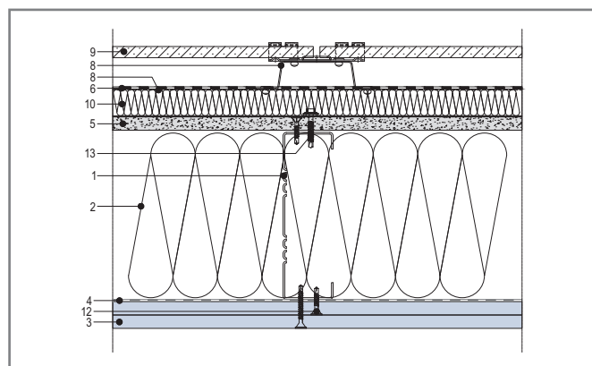
Рис. 2. Основные компоненты наружной каркасно-обшивной стены
