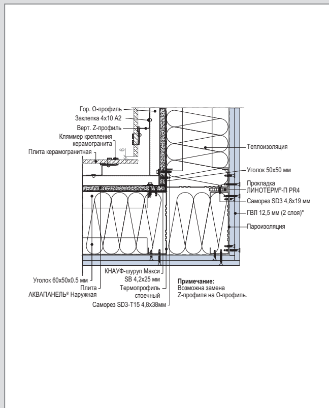
В 10 – WM 112 (2) С. Внутренний угол
