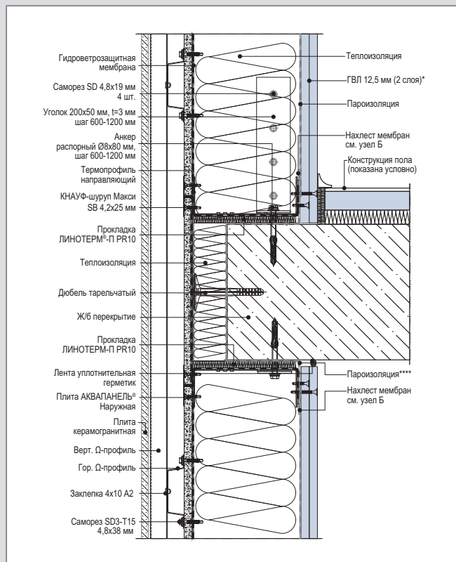
В 4 – WM 112 (2) С. Вертикальный разрез рядового модуля. Примыкание к перекрытию. Вариант 2
