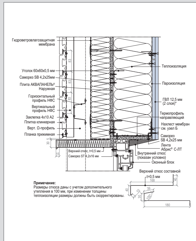
А 5 – WM 111 (4а 100) С. Верхнее примыкание к оконному блоку
