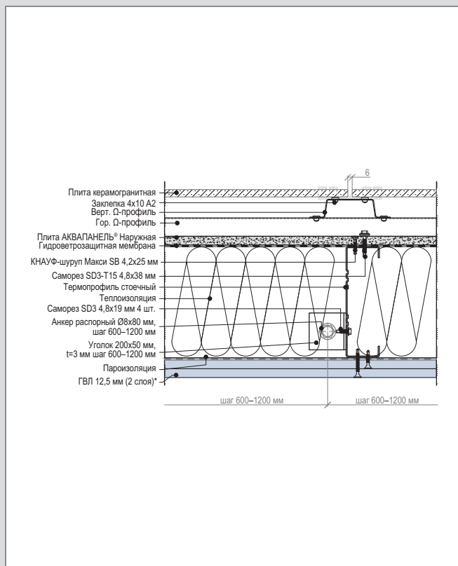
В 5 – WM 112 (2) С. Горизонтальный разрез рядового модуля. Примыкание к перекрытию. Вариант 2
