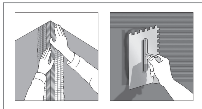
Рис. 28. Армирование углов
