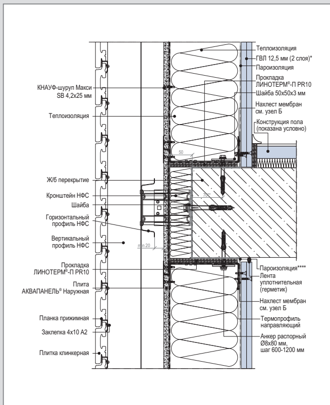
В 1 – WM 112 (2) С. Вертикальный разрез рядового модуля. Примыкание к перекрытию
