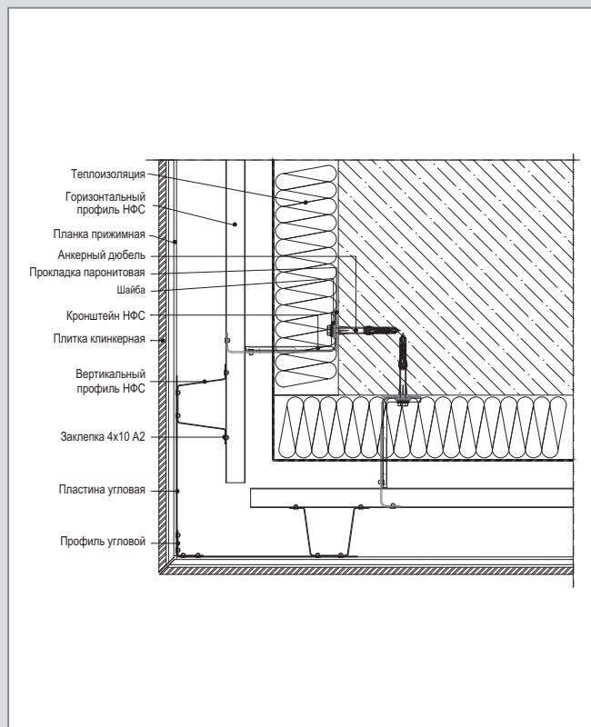
A 3 – WM 111 (4а 100) С. Горизонтальный разрез внешнего угла по перекрытию
