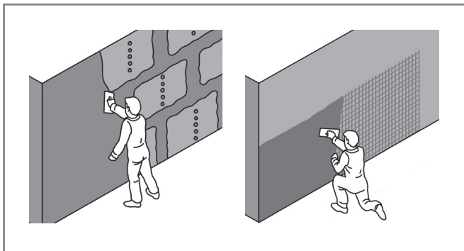
Рис. 30. Нанесение базового штукатурного слоя
