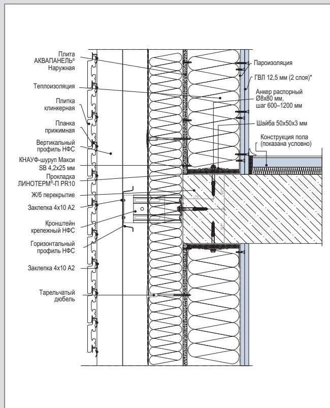
A 1 – WM 111 (4а 100) С. Вертикальный разрез рядового модуля. Примыкание к перекрытию
