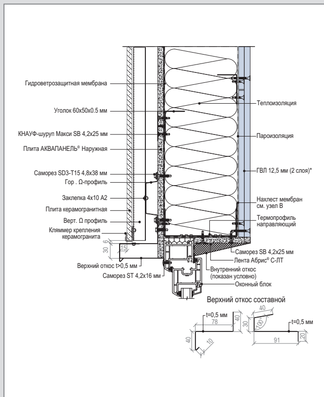
В 7 – WM 112 (2) С. Верхнее примыкание к оконному блоку
